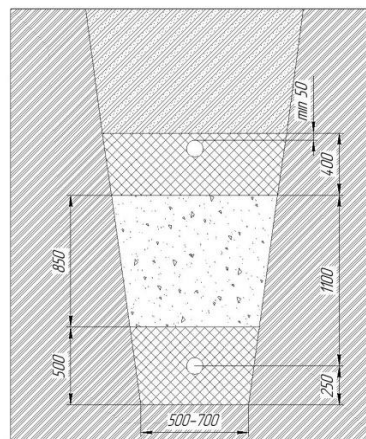
Рисунок 11 – Фильтрующая траншея
