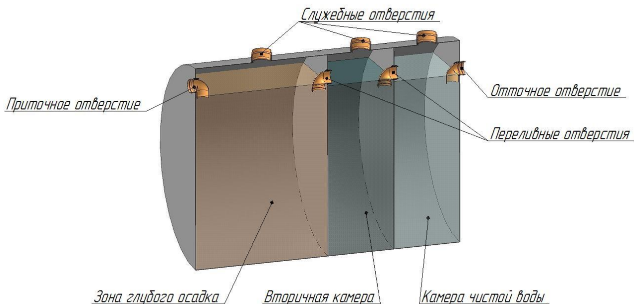
исунок 1 – Принцип работы септика SANI-S
