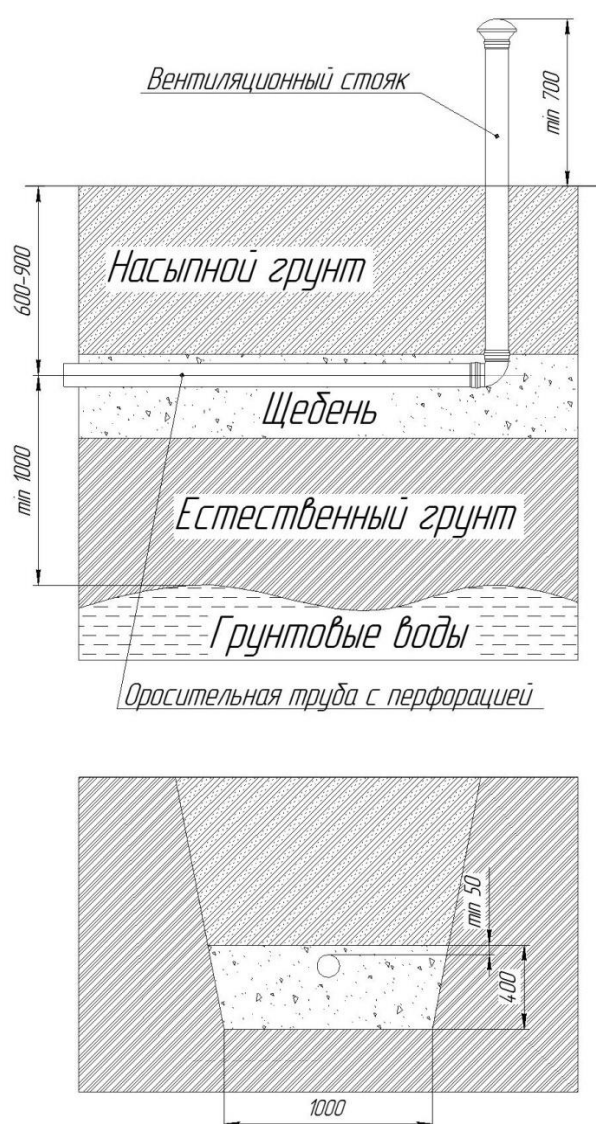
Рисунок 10 – Впитывающая траншея
