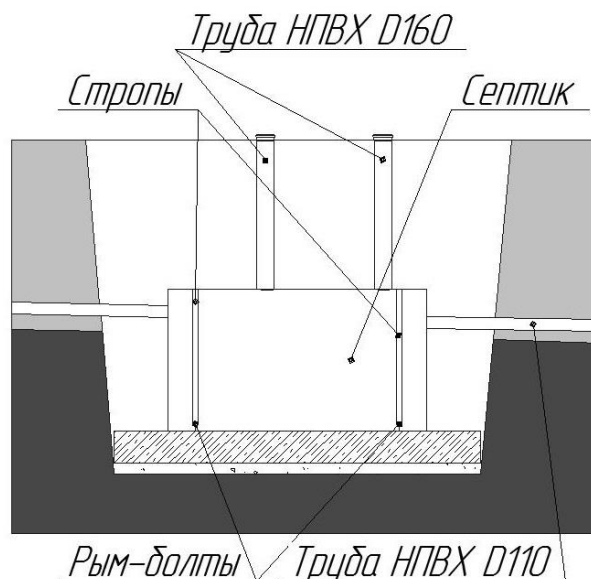
Рисунок 6 – Монтаж подводящей трассы и установки
