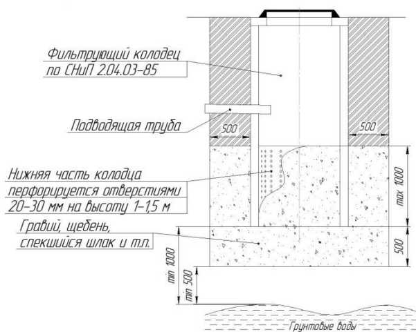
Рисунок 9 – Фильтрующий колодец
