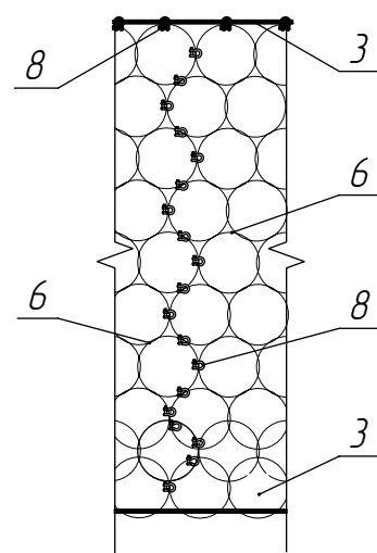
Схема соединения полотен кольчужной сети
