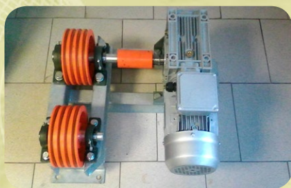
Приводная станция
