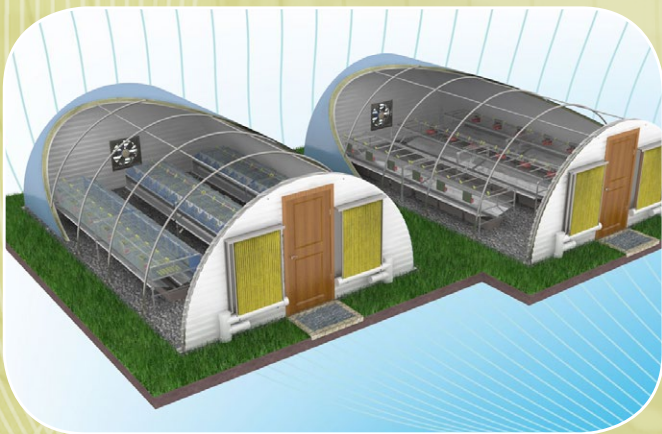
Ферма на 54 кроликоматки (6х6м)
