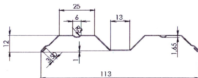
М-образный 113мм
