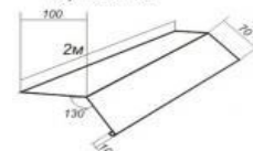
Конёк
