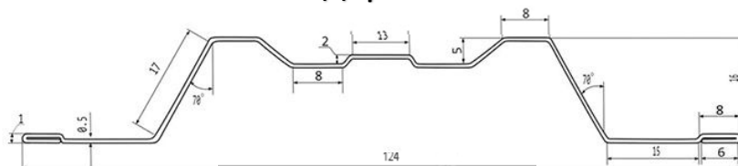
Эконом 104мм
