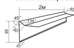
Планка "домиком"
