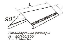
Конёк
