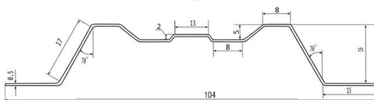
М-образный 113мм
