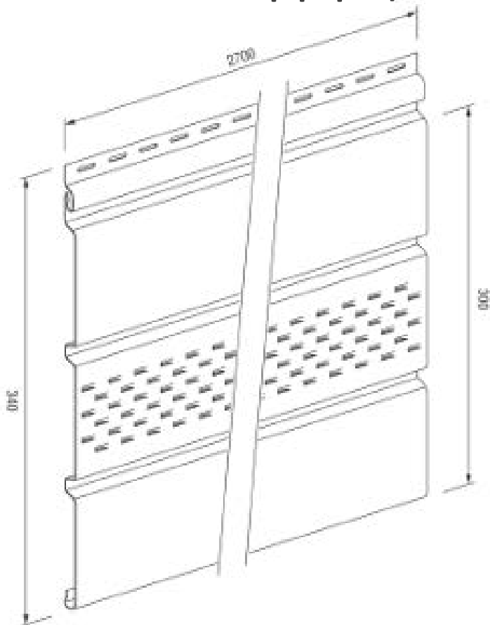
SV-07 панель с частичной перфорацией
