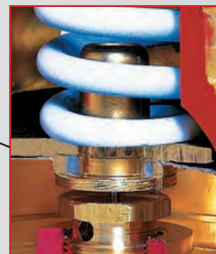
Защищенный от несанкционированных манипуляций самофиксирующийся внутренний предохранительный клапан
