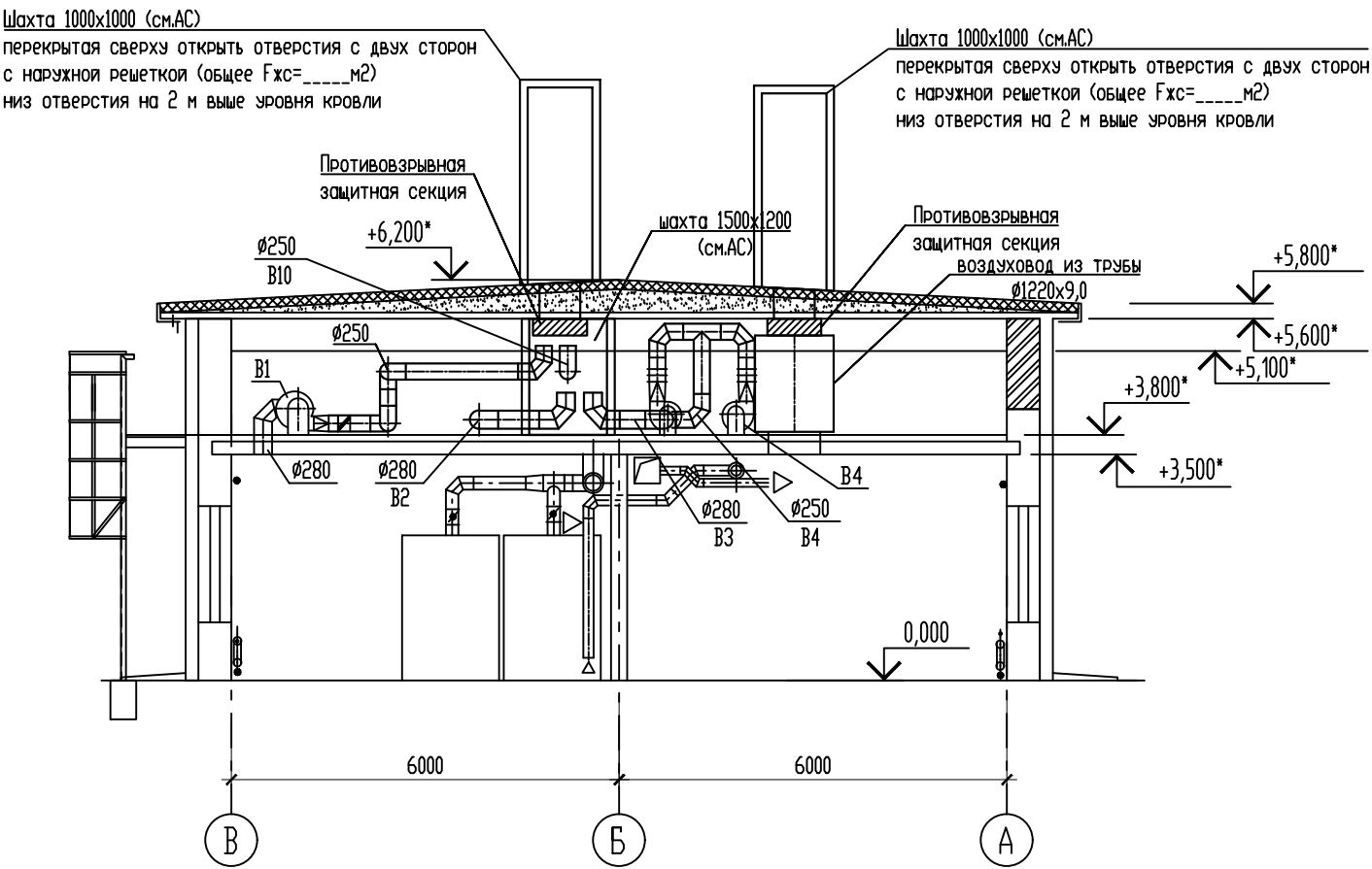
Разрез 2 - 2
