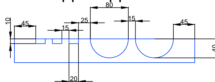
Вид сзади
