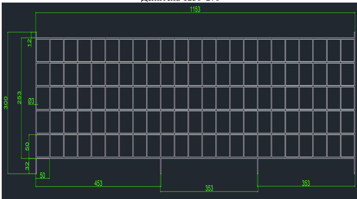
Делитель 1250*270
