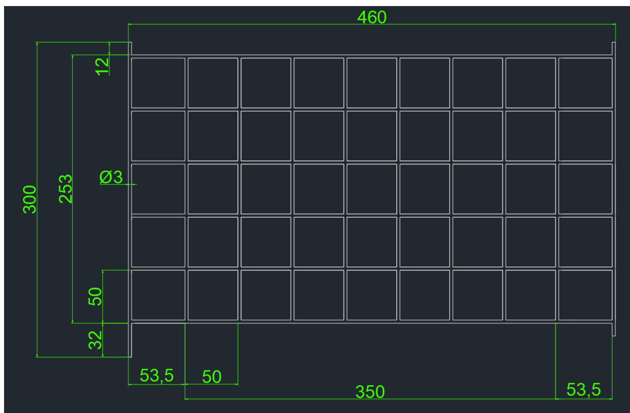
Делитель 500*270
