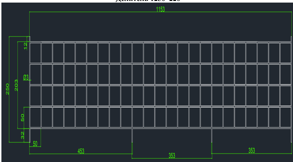
Делитель 1250*220
