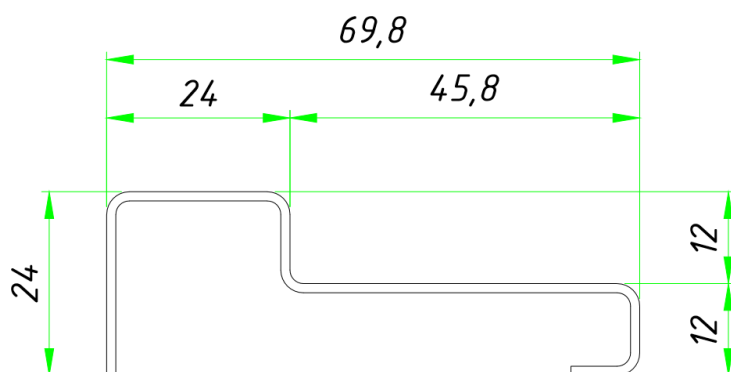
Вариант 7 Низкий порог для EIS-60
