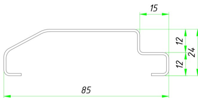
Вариант 4 Скошенный порог
