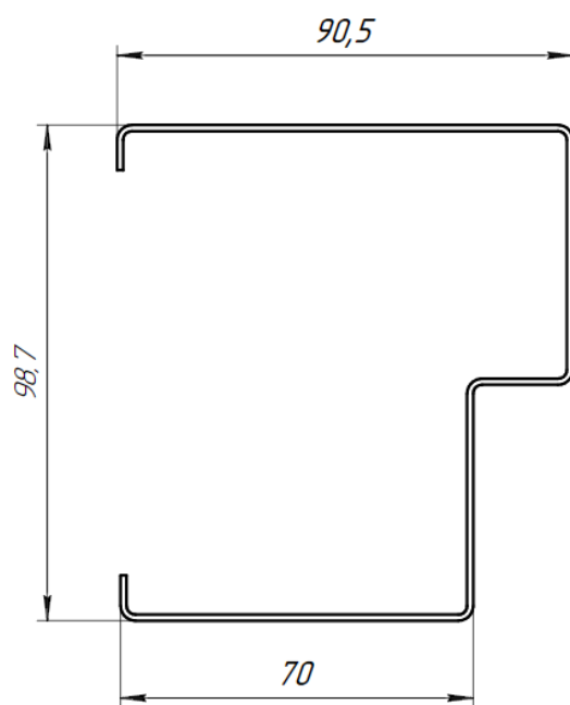
Вариант 3 Для дверных проёмов с четвертью без ОБН (282)
