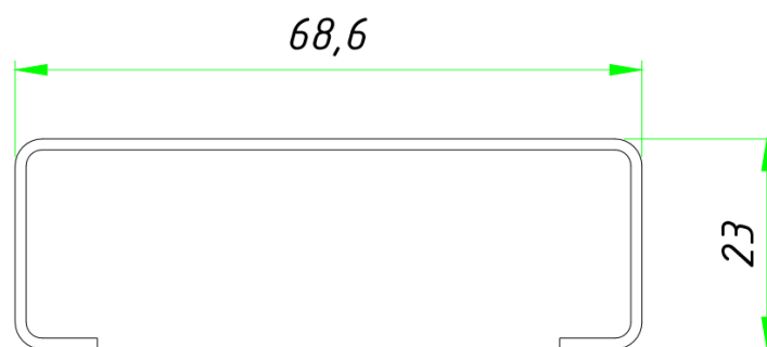
Вариант 1 Стандартный вариант
