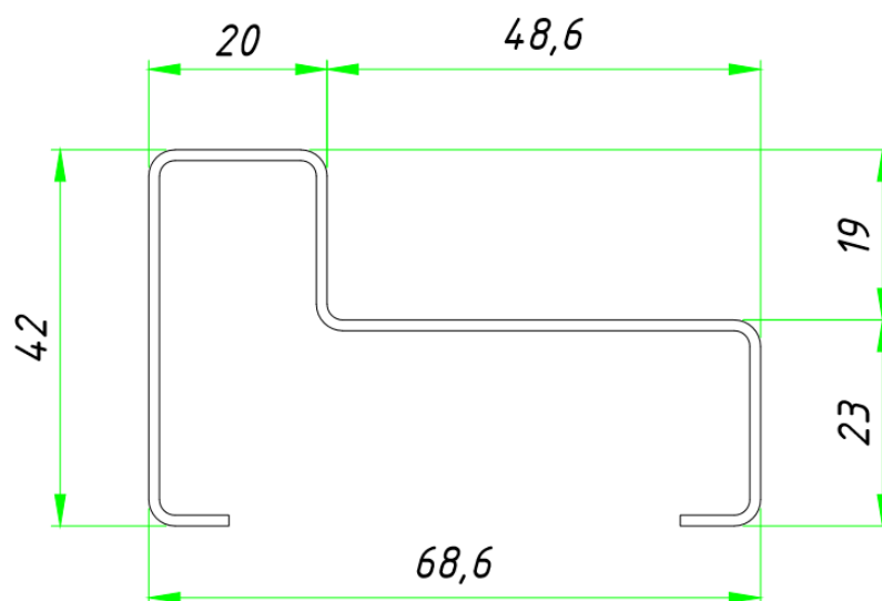
Вариант 1 Стандартный вариант
