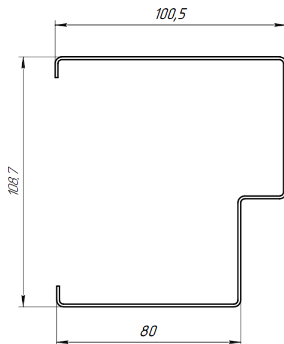
Вариант 4 Для проёмов с четвертью без ОБН (315)
