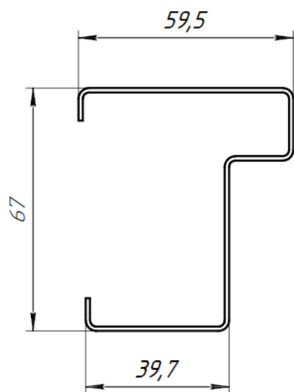
Вариант 2 Для дверей без ОБН (190, петля не выходит за край коробки)
