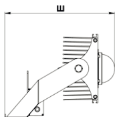
Тип КСС С, 130x30°
