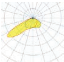
Тип КСС С, 130x30°
