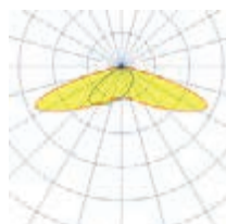
Тип КСС ШБ, 155x70°
