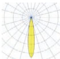
Тип КСС К, 12°
