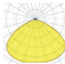
Тип КСС Д, 120°
