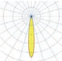
Тип КСС К, 15°
