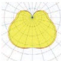
Тип КСС М
