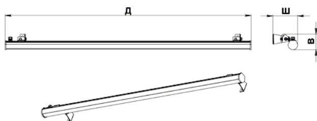
Тип КСС Д, 120x210°
