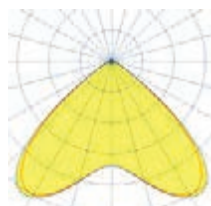
Тип КСС Л, 90°
