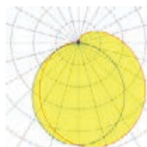
Тип КСС Д, 135°
