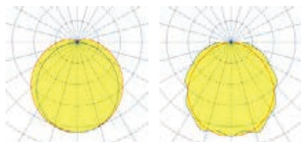
Тип КСС Д, 135°
