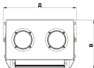
Тип КСС ШБ, 140x85°
