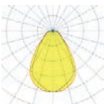
Тип КСС Д, 75°
