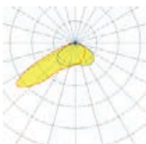
Тип КСС Г, 130x30°
