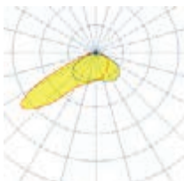
Тип КСС С, 130x30°
