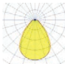
Тип КСС Д, 80°
