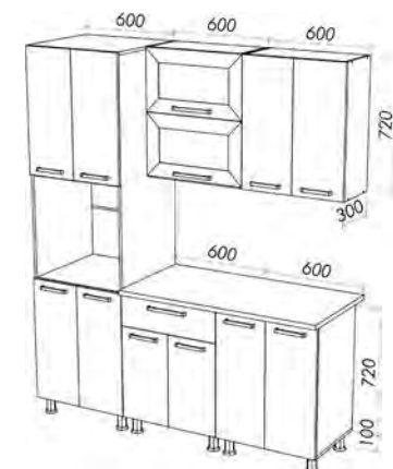
«Дельта 9» 2140x1800x600 мм.
