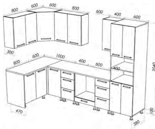
«Дельта 5» 2140x3400x2200 мм.
