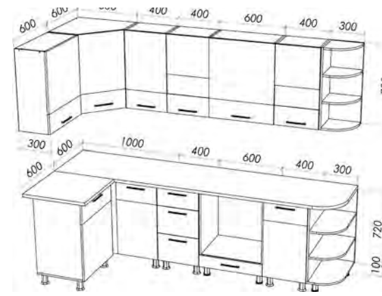
«Николь 9» 2140x1200x2700 мм.
