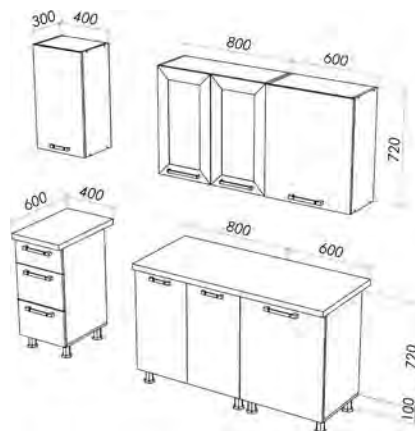
«Дельта 14» 2140x2000x600 мм.
