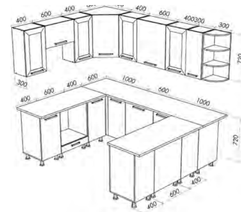
«Дельта 8» 2140x2600x600 мм.
