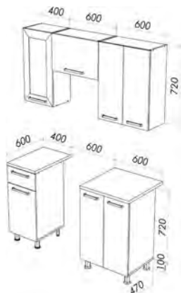
«Дельта 12» 2140x1800x600 мм.
