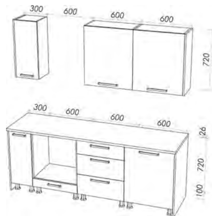
«Дельта 2» 2140x2400x600 мм.
