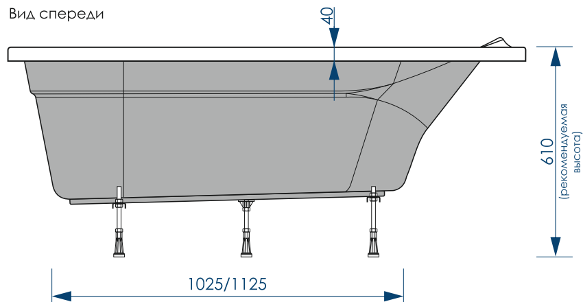
Вид спереди
