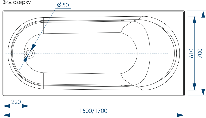
Вид сверху
