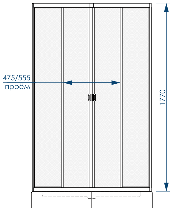
Вид спереди
