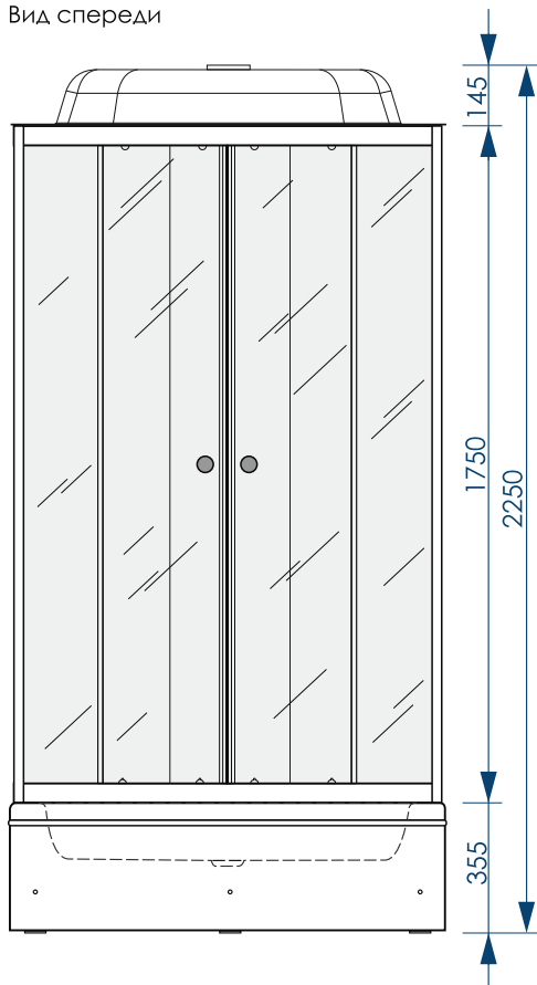
Вид спереди
