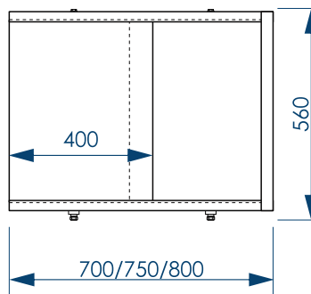
Торцевой экран. Вид спереди
