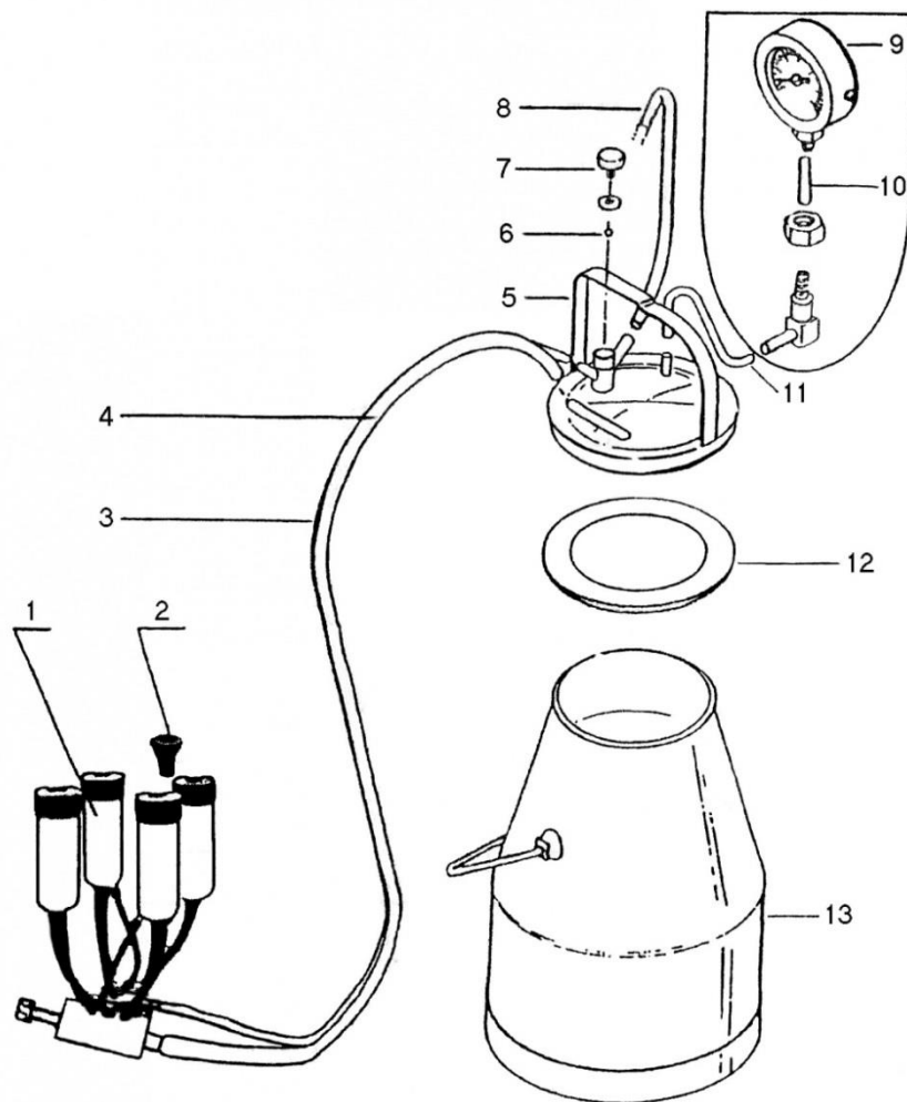
Монтажная схема №1
