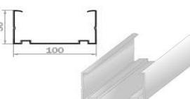
Профиль стоечный ПС 100 x 50
