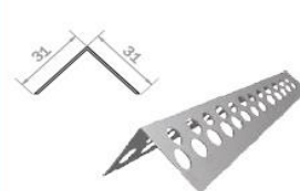
Профиль углозащитный ПУ 31 x 31
