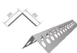
Профиль углозащитный ПУ 20 x 20
