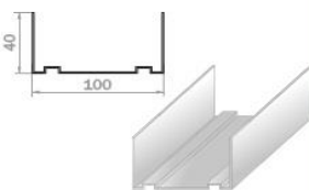
Профиль направляющий ПН 100 x 40
