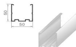
Профиль стоечный ПС 50 x 50
