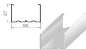
Профиль потолочный ПП 60 x 27
