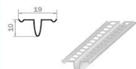
Профиль маячковый ПМ 10 мм
