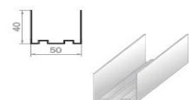
Профиль направляющий ПН 50 x 40
