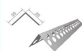
Профиль углозащитный ПУ 25 x 25
