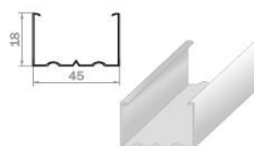
Профиль потолочный "Эконом" ПП 45 x 18
