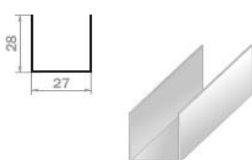
Профиль потолочный направляющий ППН 28 x 27
