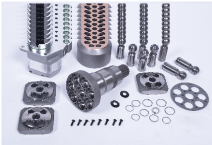
Model:A7V0107
