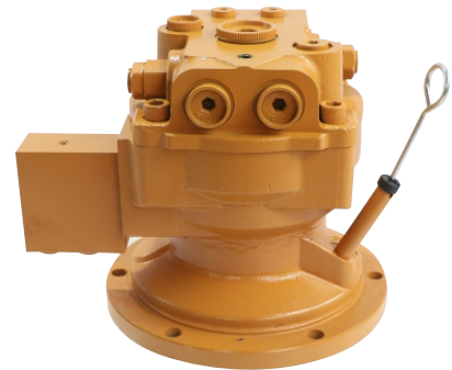
Model:DH60(JMF29)
